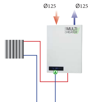
Käyttövesi ja talon lämmitys minkä tahansa lämmönlähteen rinnalla (vaihtoventtiili optiona).
