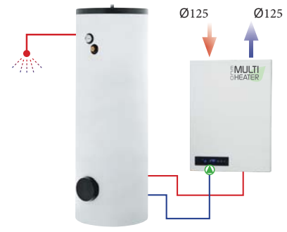
Suora kytkentä käyttövesivaraajaan.
